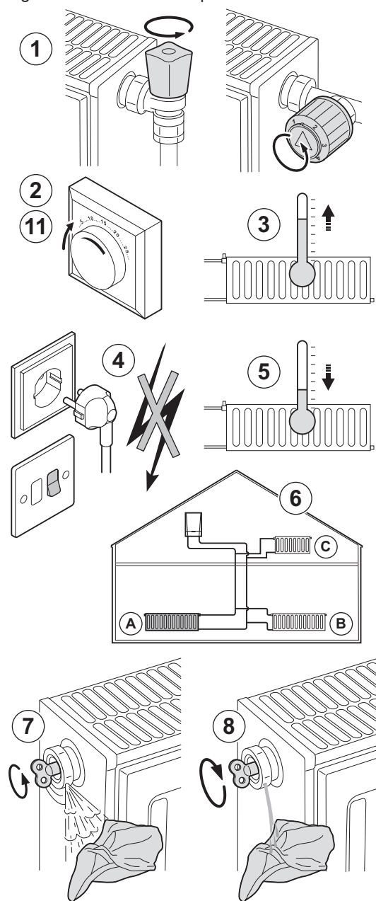
Fig.51 Deareazione impianto
