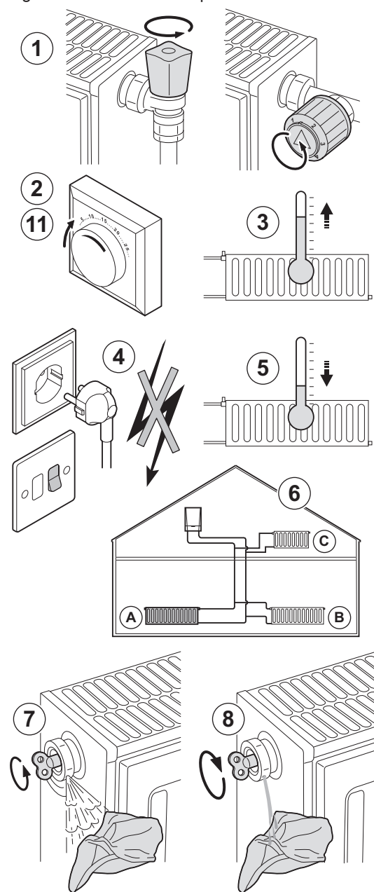
Fig.51 Deareazione impianto
